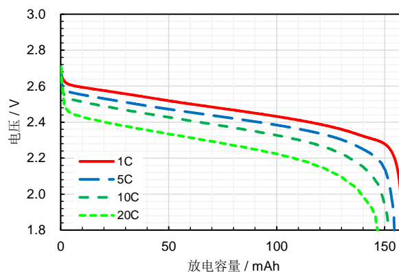
放电特性
