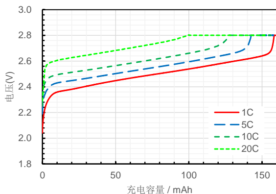
充电特性
